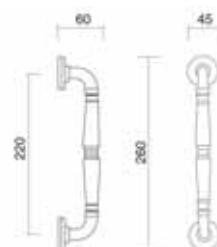
Art. 0035 Maniglione Mod.800 Pull handle Mod.800
